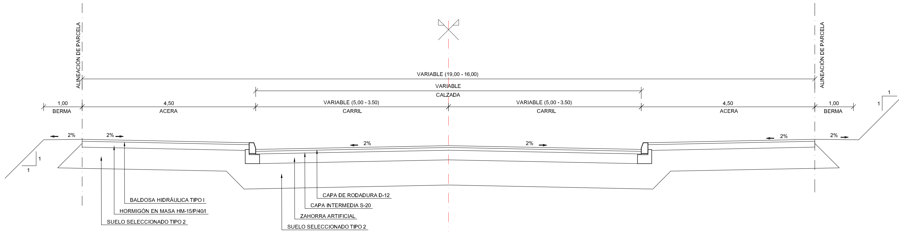
VIAL 1 (DEL PK 0+000 AL PK 0+090)
