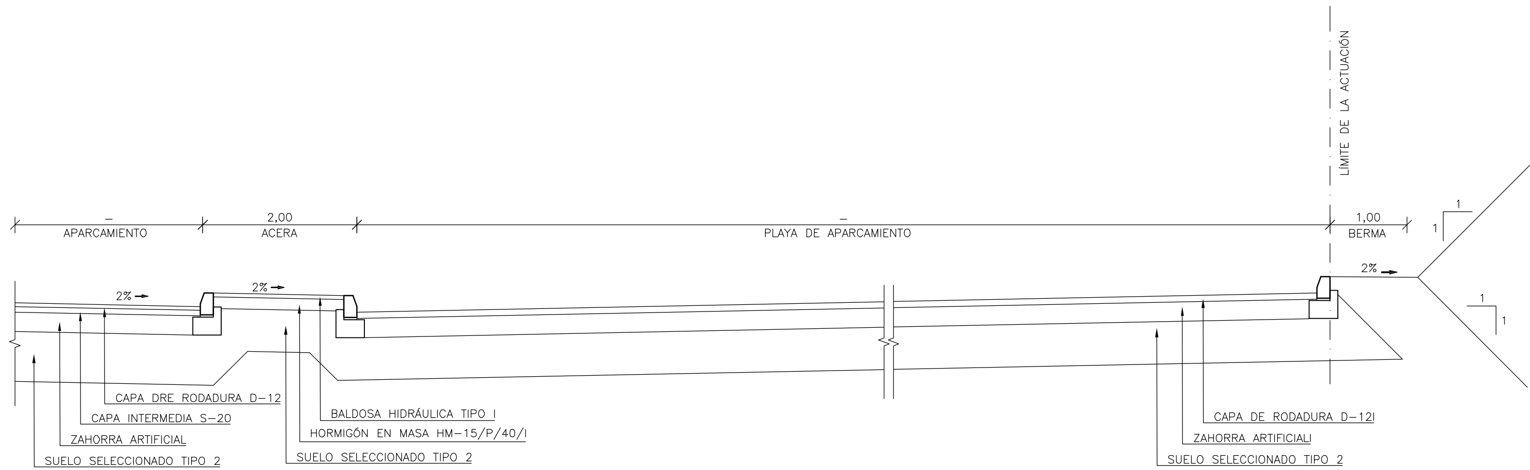
PLAYAS DE APARCAMIENTO ESCALA 1:50
