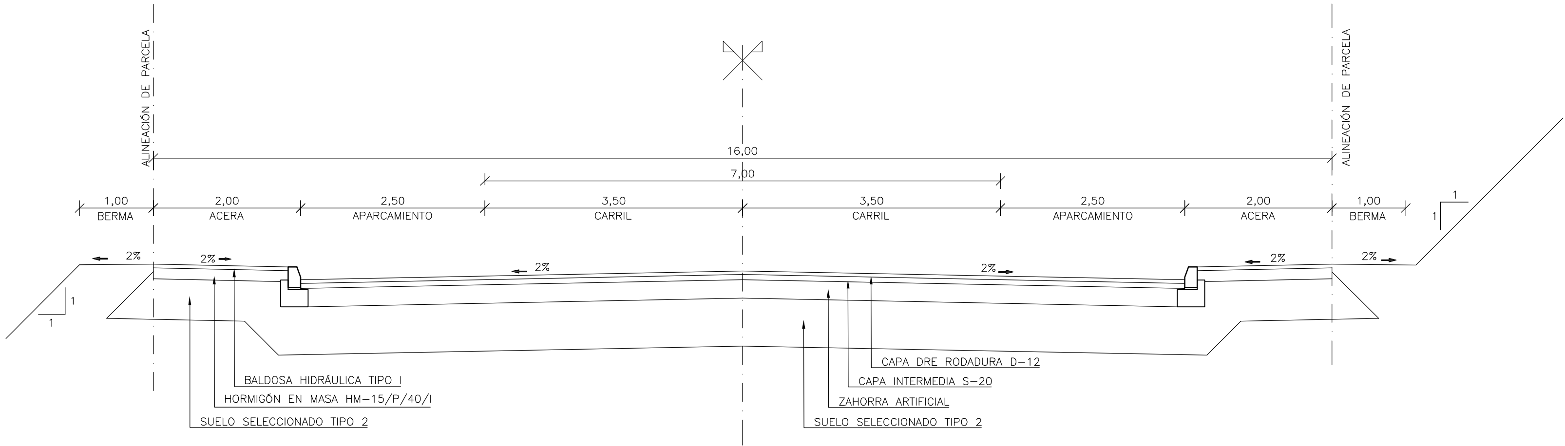
RESTO DE VIALES ESCALA 1:50
