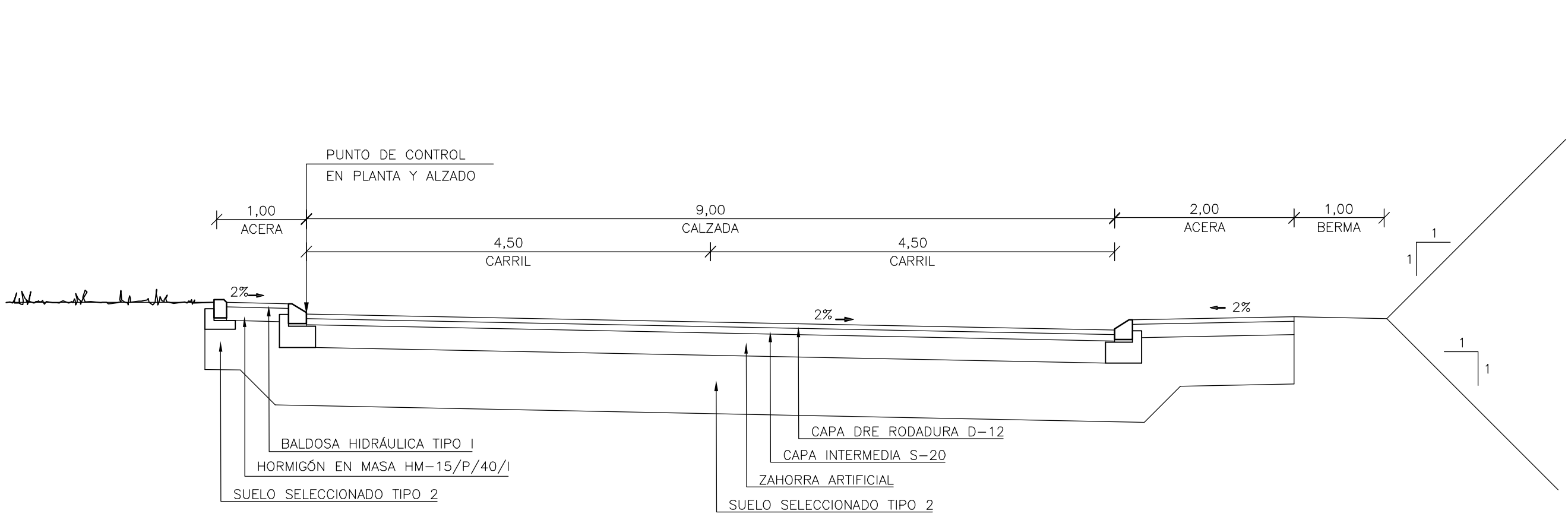
GLORIETAS EJES 7 Y 8 ESCALA 1:50
