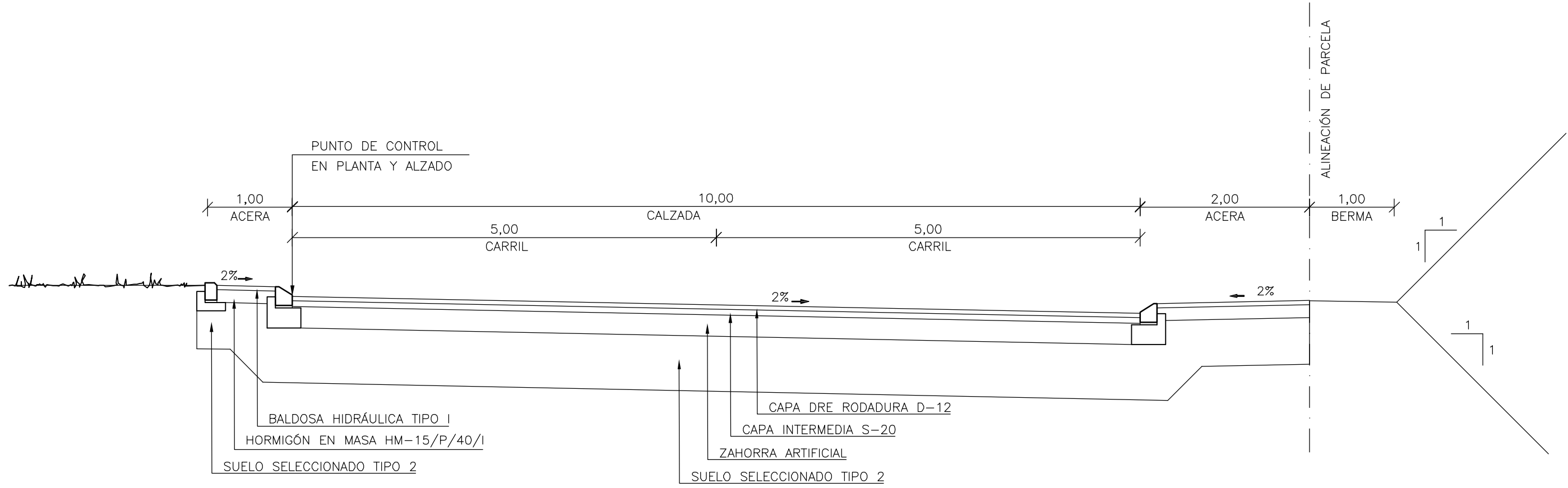
GLORIETA EJE 9 ESCALA 1:50
